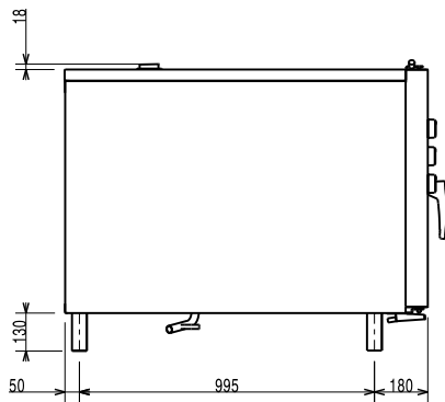
Oldalnézet
